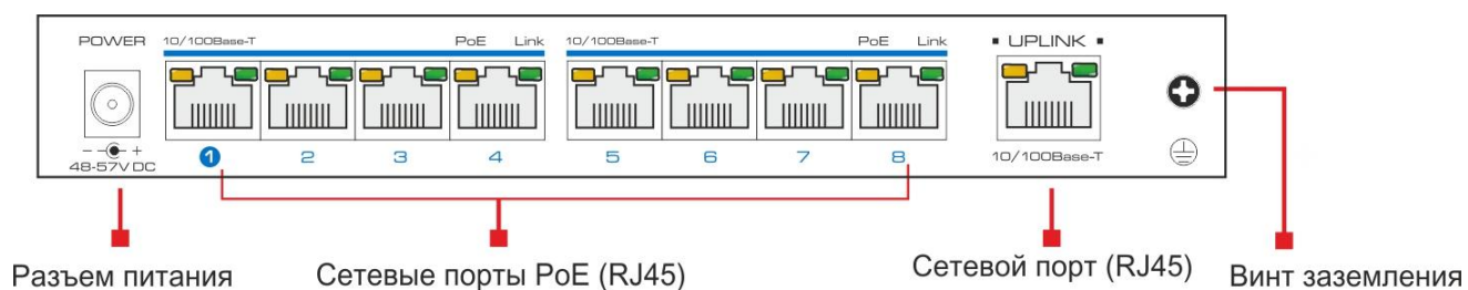
Рис. 1 Задняя панель коммутатора
